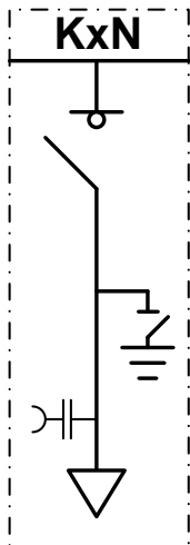
KxN = Interrupteur
